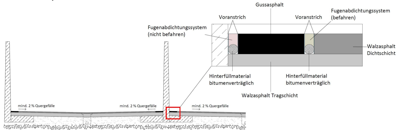
Abb. 6: Asphalt - Betonfertigteile (gerade Wand) mit Ortbetonfuß
