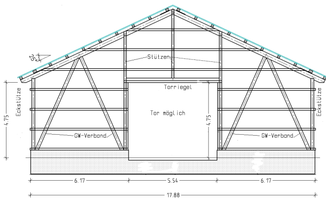
Schnitt Giebelwand
