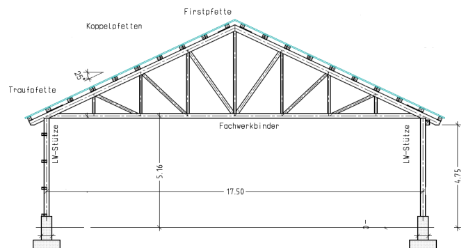
Hallen-Querschnitt
