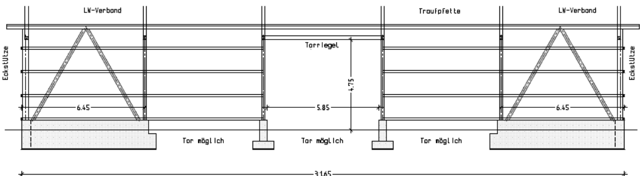
Schnitt Längswand
