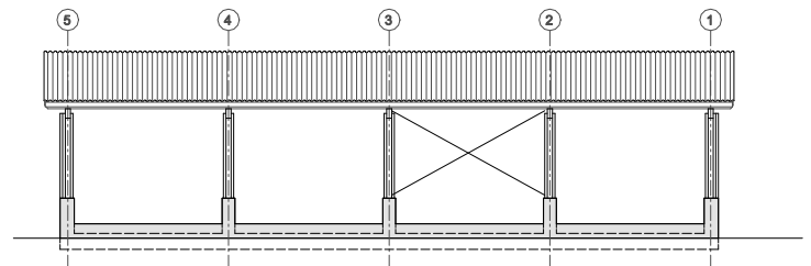
Ansicht Traufseite
