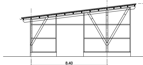
Ansicht Giebelseite mit Ausriegelung für Fassade
