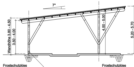
Schnitt
