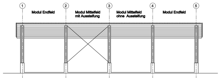
Ansicht Firstseite
