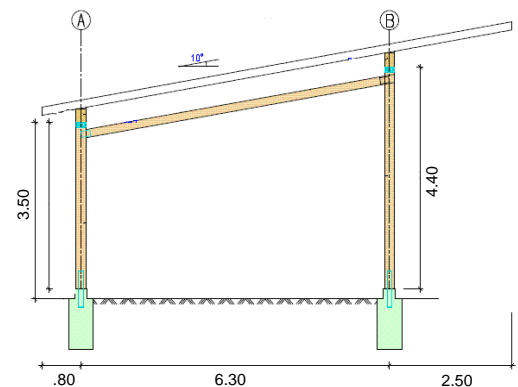
Schnitt D - D: Mittelfeld
