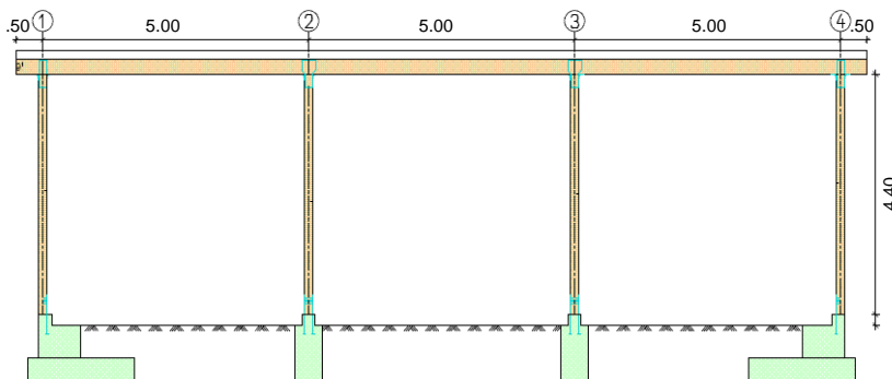
Schnitt B - B: Längswand vorne
