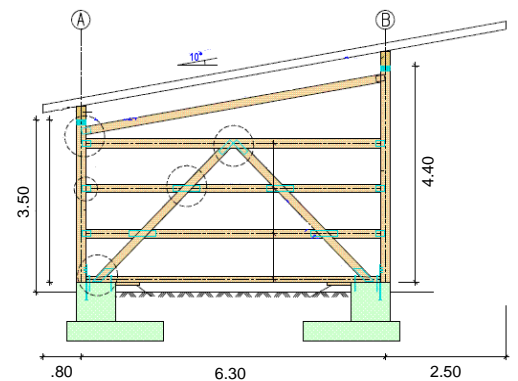
Schnitt A - A: Giebelwand
