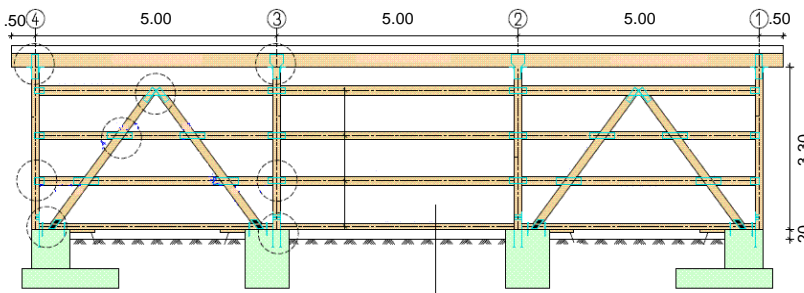
Offenes Mittelfeld möglich ohne Querriegel
