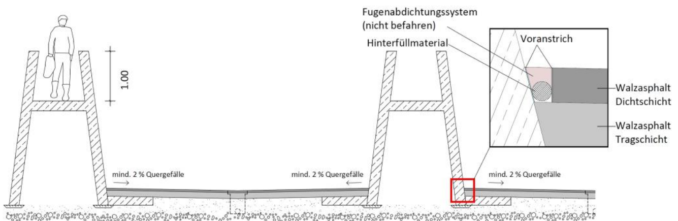
Abb. 12: Asphalt - Betonfertigteil begehbar (schräge Wand)
