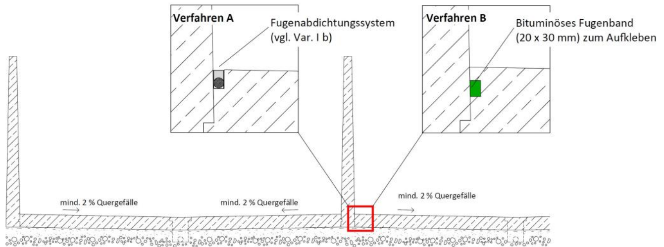
Abb. 4: Ortbeton - Betonfertigteil (gerade Wand)
