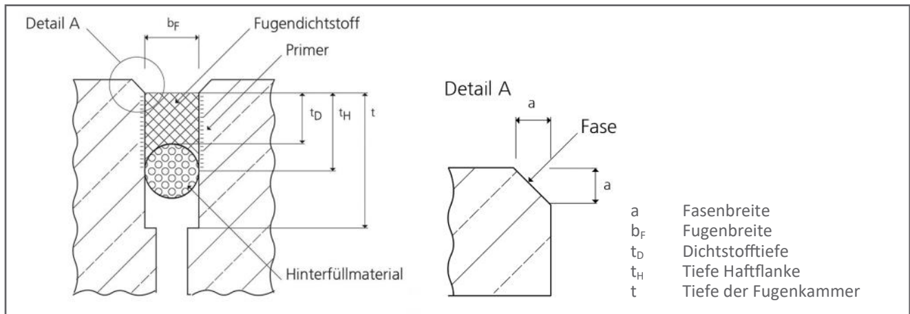
Abb. 1 : Detail Fugenabdichtung mit Fugendichtstoff (Quelle: verändert nach Saba)
