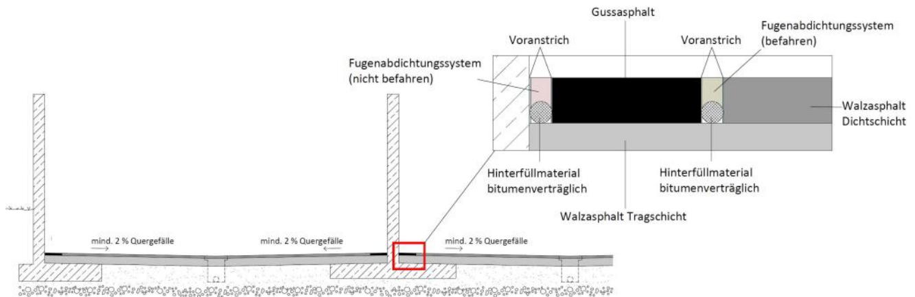
Abb. 5: Asphalt - Ortbeton (gerade Wand)
