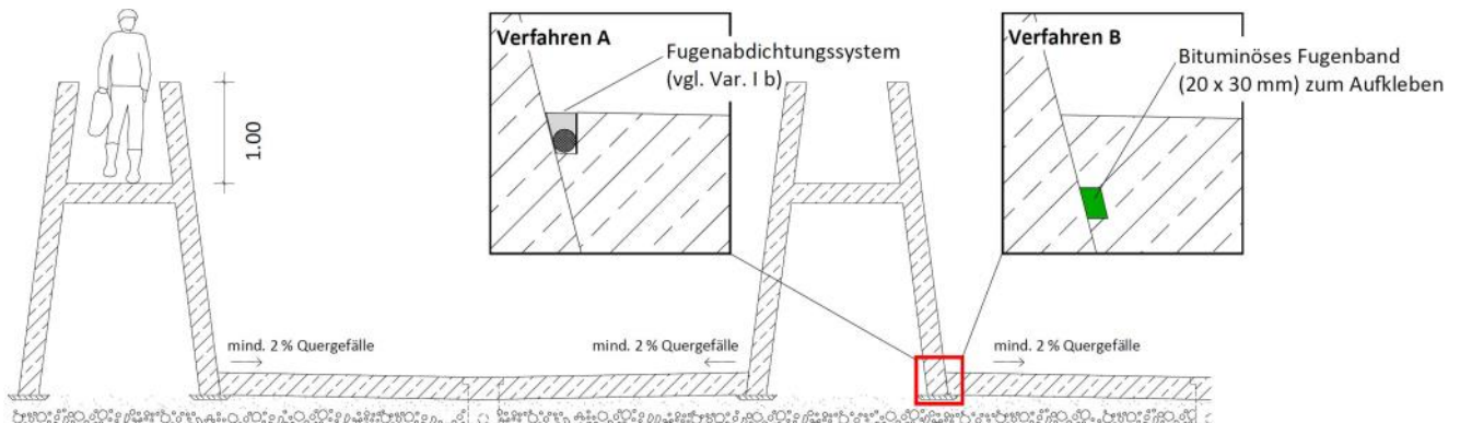
Abb. 11: Ortbeton - Betonfertigteil begehbar (schräge Wand)
