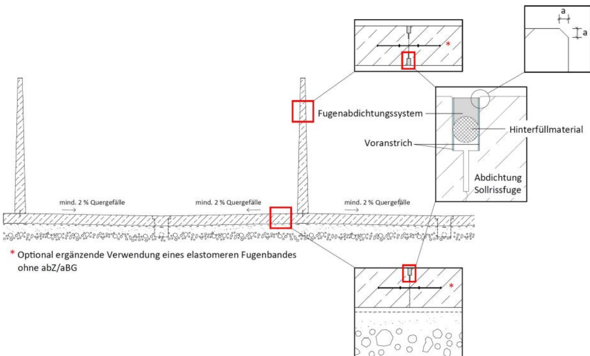
Abb. 3: Ortbeton - Ortbeton (gerade Wand) - Verwendung von Fugendichtstoffen im Rahmen der abZ/aBG (siehe auch Kapitel 6.2)
