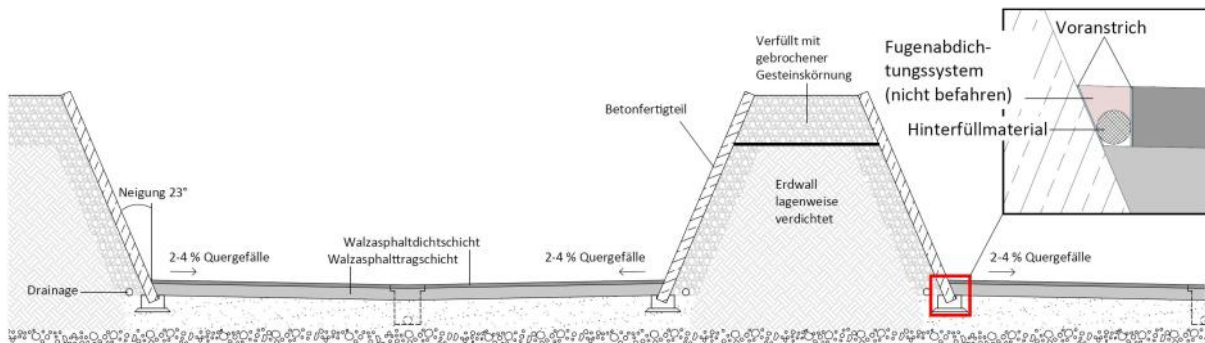
Abb. 10: Asphalt - Betonfertigteil (Traunsteiner Wand); weitere Details siehe abZ/aBG, Anlage 1 - 6
