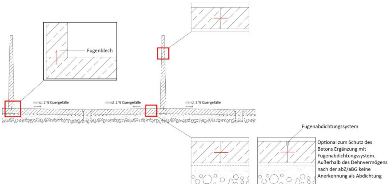
Abb. 2: Ortbeton - Ortbeton (gerade Wand) - Verwendung von Fugenblechen (siehe auch Kapitel 6.1)
