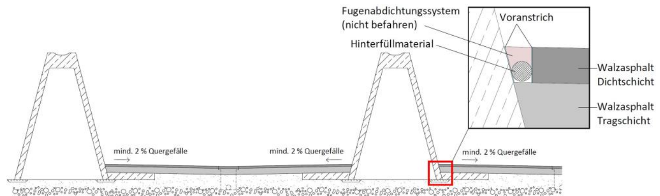
Abb. 8: Asphalt - Betonfertigteil (schräge Wand)
