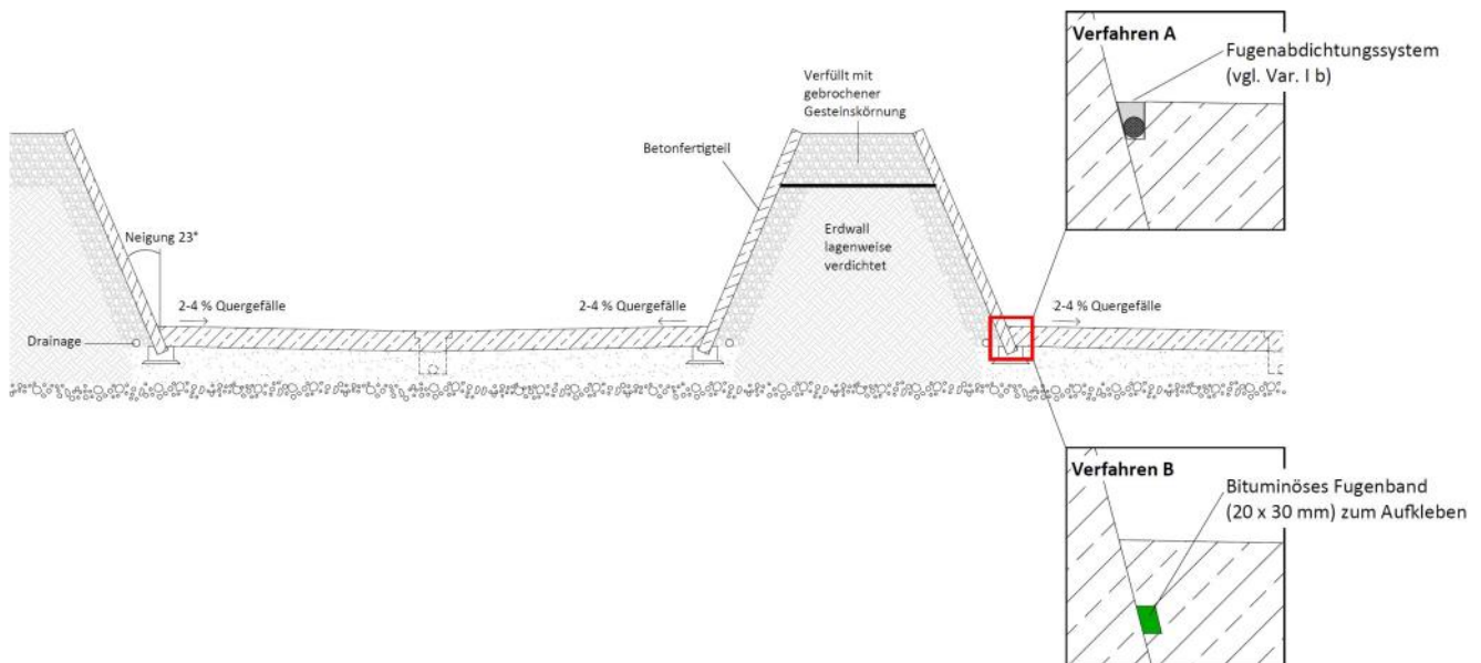
Abb. 9: Ortbeton - Betonfertigteil (Traunsteiner Wand); weitere Details siehe abZ/aBG, Anlage 1 - 6
