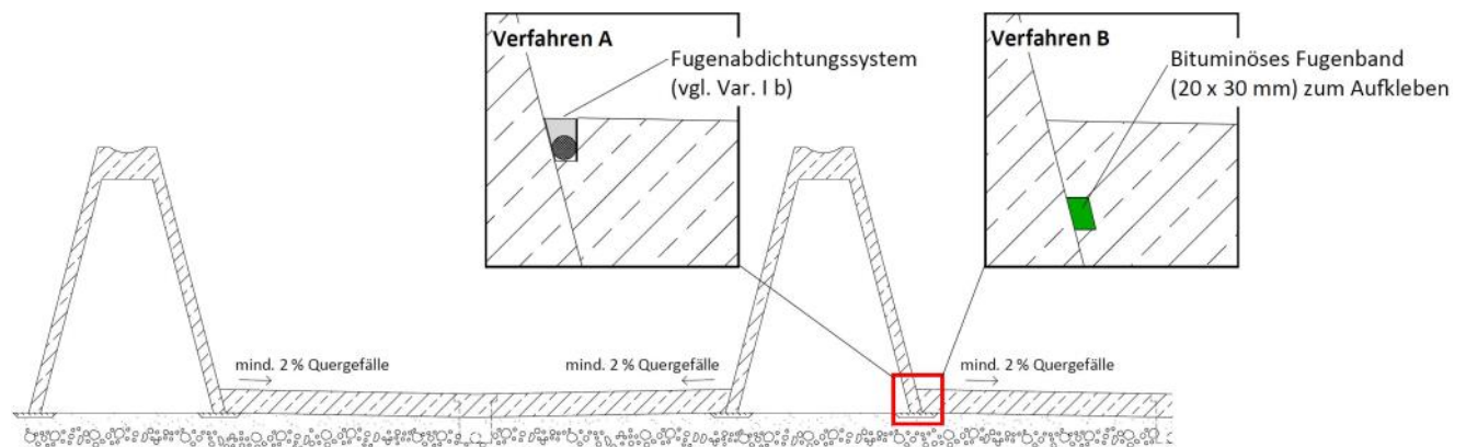
Abb. 7: Ortbeton - Betonfertigteil (schräge Wand)
