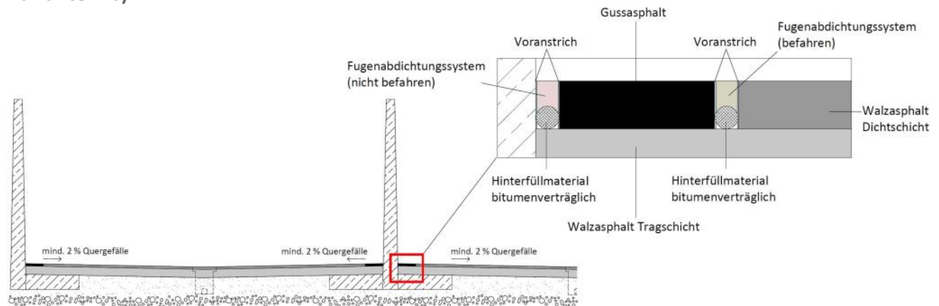
Abb. 6: Asphalt - Betonfertigteil (gerade Wand) mit Ortbetonfuß
